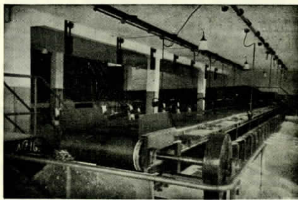
Jälkivuolijain työpöytä, liukuhihna, mistä puhtaat puut siirtyvät alla olevaa hihnaa pitkin tehtaalle.
