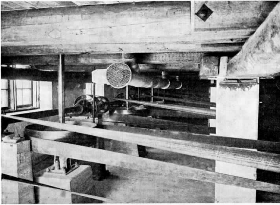
Kuva 6. Myllykoneiston välivaihteita.
