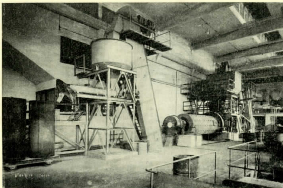
Karbidin jauhetta pölyksi putkimyllyllä ja johdetaan typetysastioihin.
