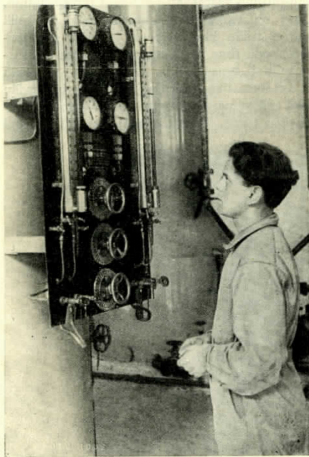
Ilman nesteyttämiskoneita.
