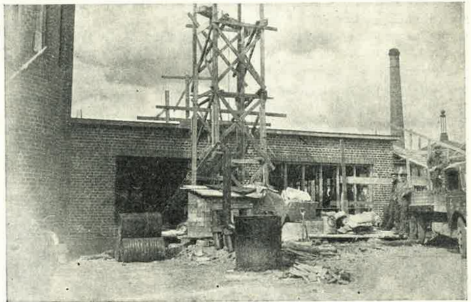
Uuden osan 3. kerros näkyy tässä.
