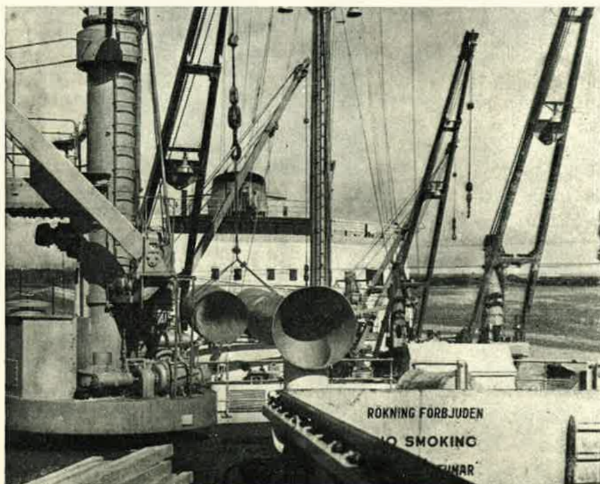
Näkymä "Los Angelesin" kannelta. Kuten huomataan, on laivassa omat nostoranansa, 7 kummallakin laidalla eli yhteensä 14.
