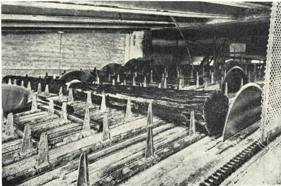
Kuva 2. Puiden katkominen 1 m:n pituisiksi pölleiksi.
