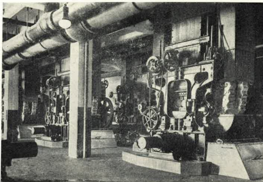
Kuva 8. Voithin kestopöytähiomakoneita, joissa hiominen tapahtuu.
