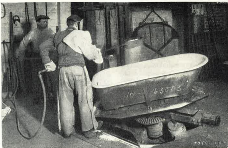
Kylpyammeen emaljointi paineilmasirottimella.
