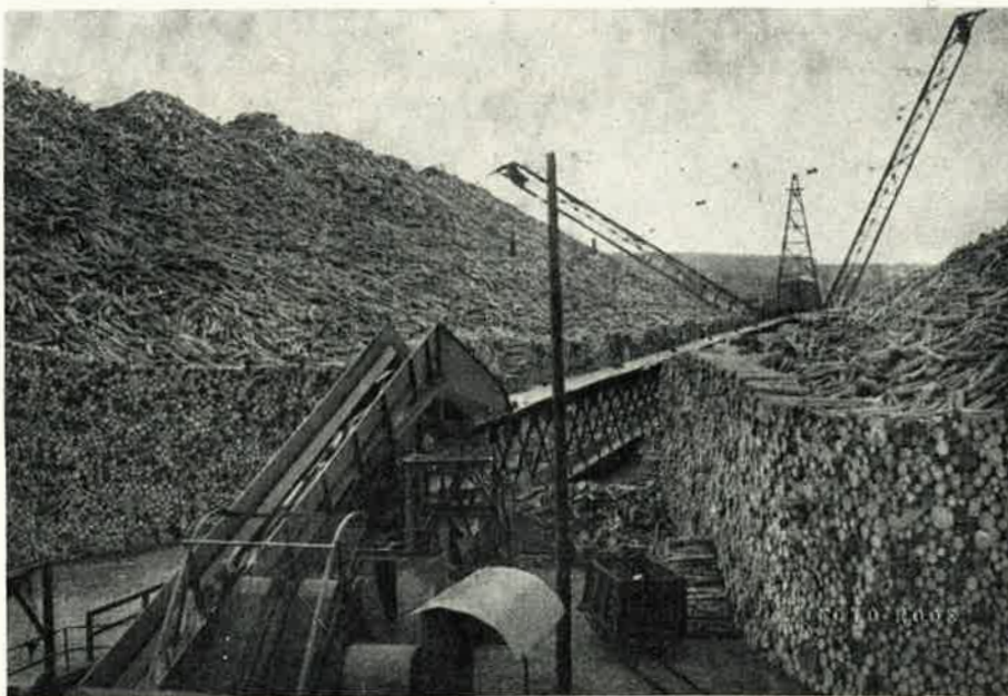
Kuva 5. Osa varastoa kuljetuslaitteineen.
