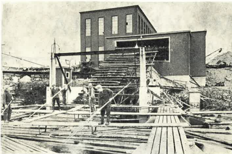
Kuva 1. Puiden syöttö puuhiomon kuorimon nostolaitteelle.
