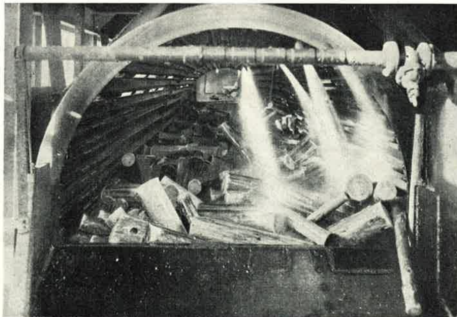
Kuva 3. Pöllejä kuorimarummussa, josta poistuessaan ne pestään voimakkailla vesisuihkuilla.
