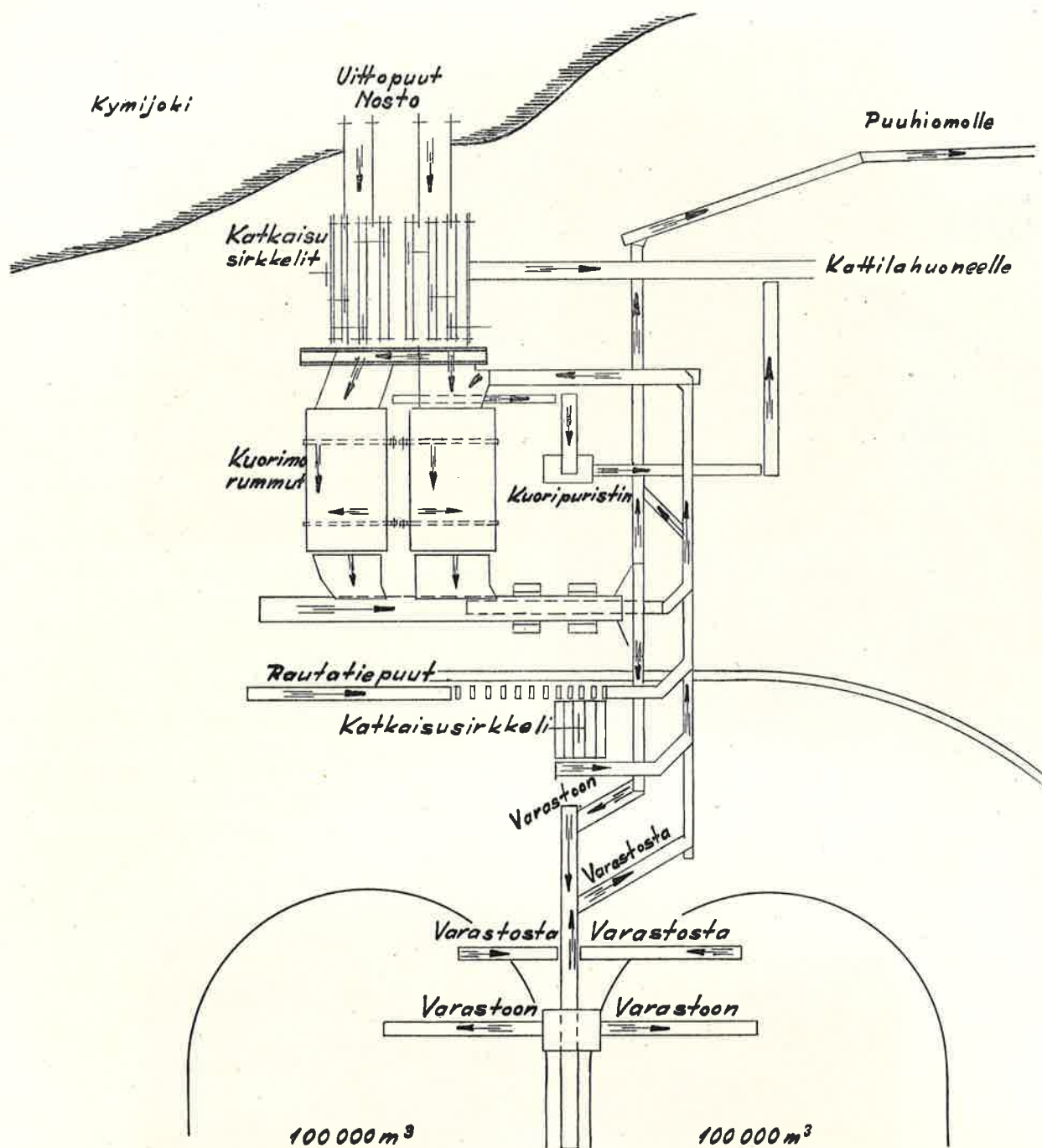
Kaaviopiiirros puiden kulusta kuorimossa ja varastoalueella.
