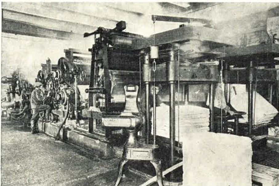
Kuva 12. Kamyrkone, jossa puuhioke paalataan myyntiä varten.
