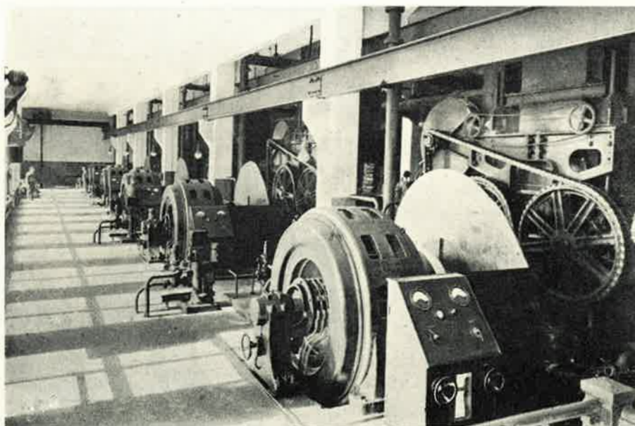
Kuva 9. 1000 hv:n sähkömoottoreita hiomakoneineen.
