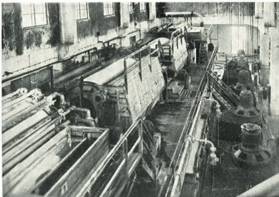
Kuva n:o 5. Imusuodattimia valkaisuosastolla. Oikealla hypokloriittivalkaisu- tornien sekoittajamoottorit.
