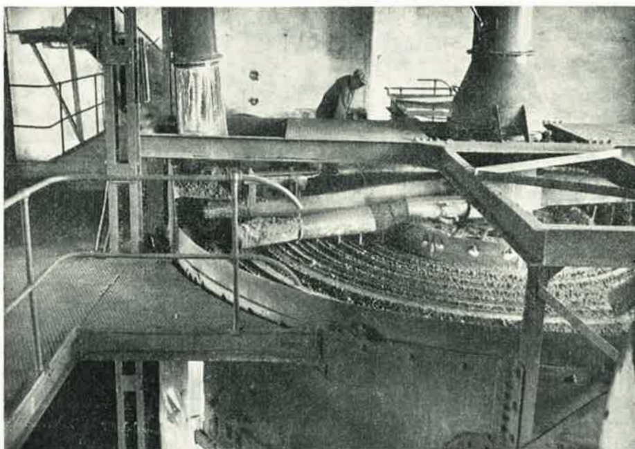
Kuva n:o 3. Kiisu-uunin yläosa.
