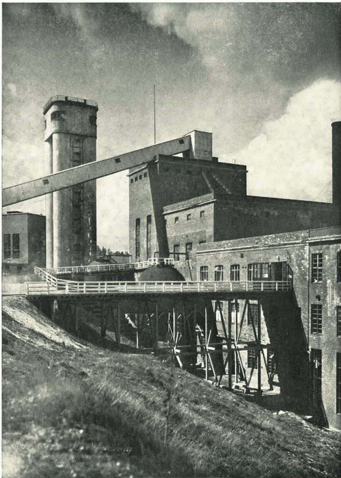
Kymin Selluloosatehtaan happotornit ja keitto-osasto.
