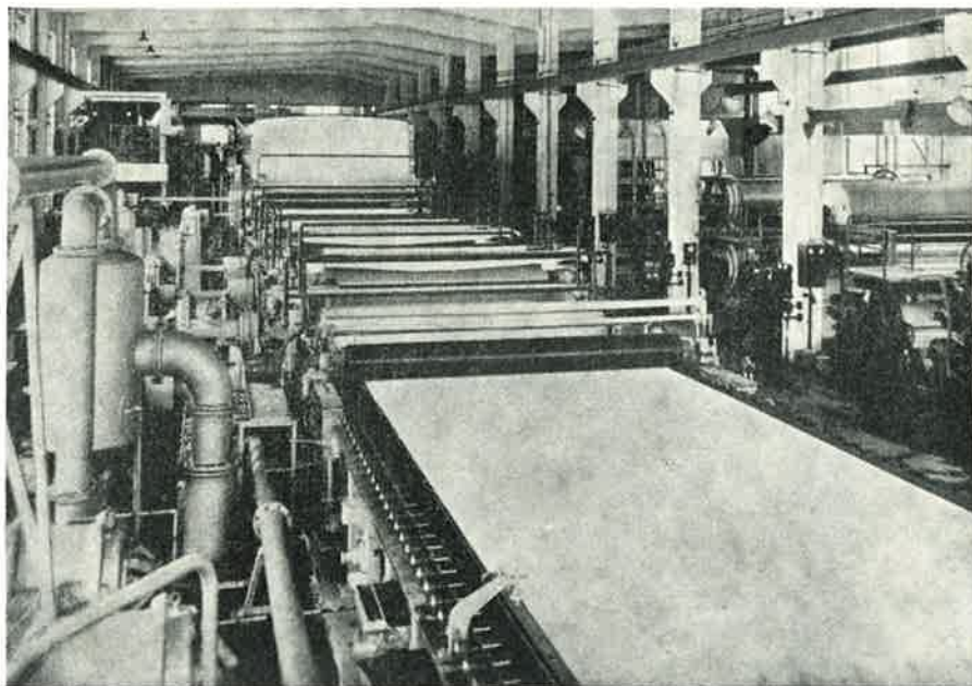
Kuva n:o 7. Kuivauskonesali. Keskellä Mintonkone, oikealla puhallinkuivaaja.
