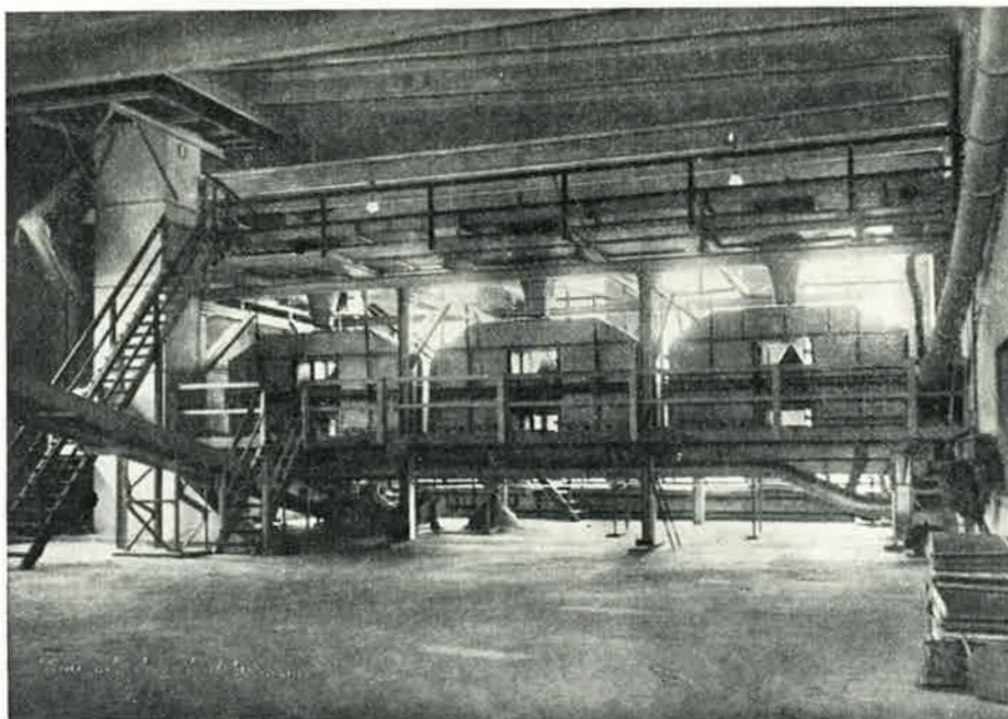
Kuva n:o 2. Kuorimon lastuseulat.
