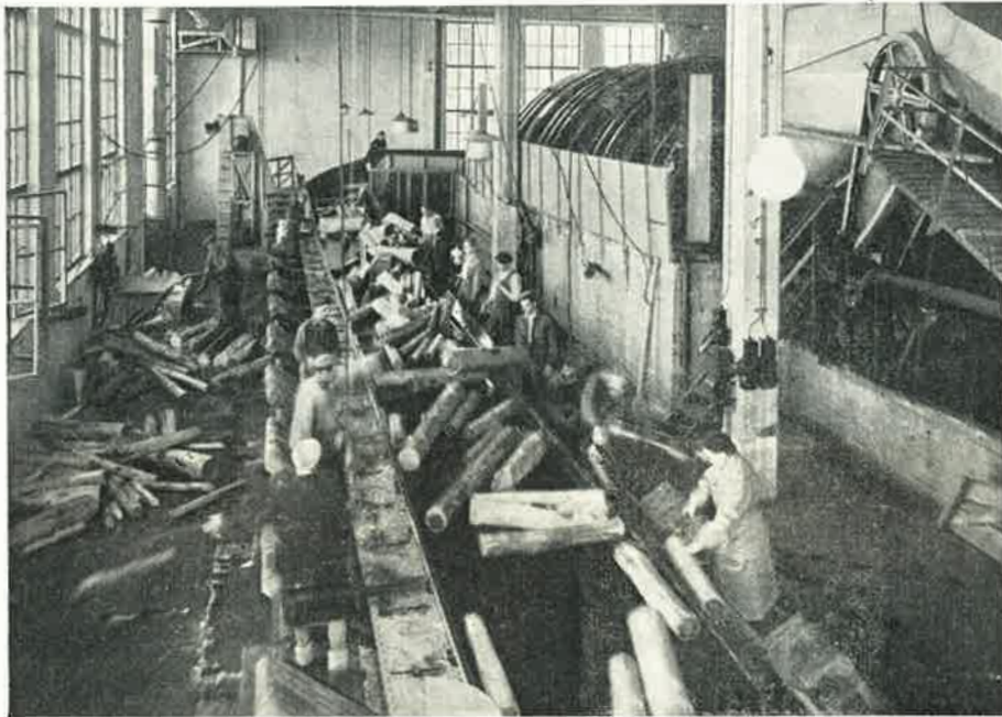
Kuva n:o 1. Kuorimon lajittelupöytä. Taustalla oikealla yksi kuorimarumpu.
