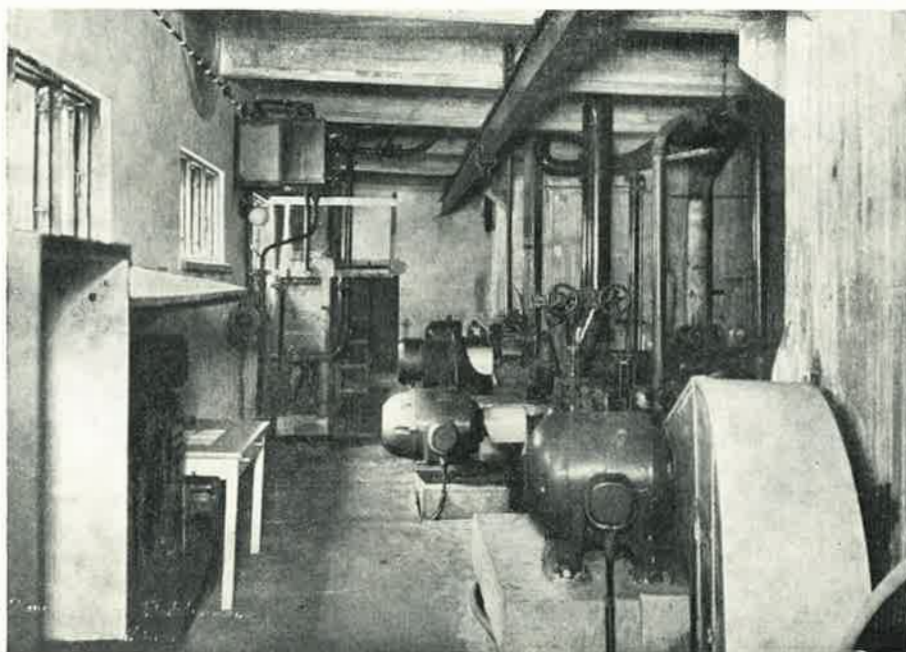
Kuva n:o 6. Valkaistun massan varastosäiliöiden pumppuhuone. Keskellä kuivaukskoneille ja paperitehtaalle pumppuavat pumput.
