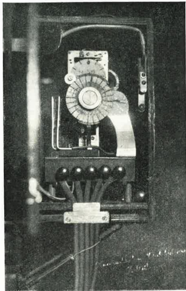
Tästä "kellosta" voi säätää laitteiden toimimisajat.
