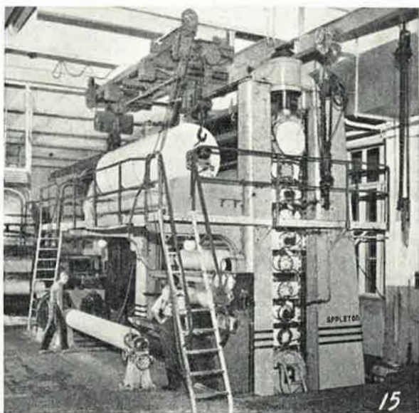
Neljännän koneen kiilloituskalanteri. Arvi Liimatainen tikapuiden takana, Matti Korpi rullan vieressä.
