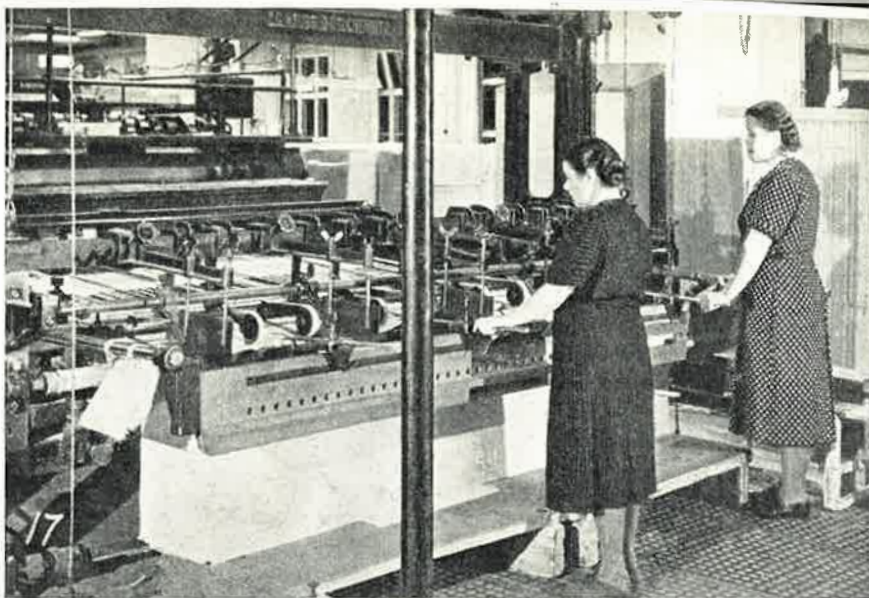
Haubold-leikkuukone. Lyyli Väkevä ja Sointu Sinkko tarkastavat koneen tekemää työtä.
