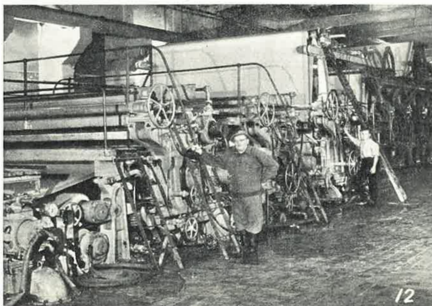
PK 6. Taavi Kataja ja Reijo Luomala koneen märässä päässä.
