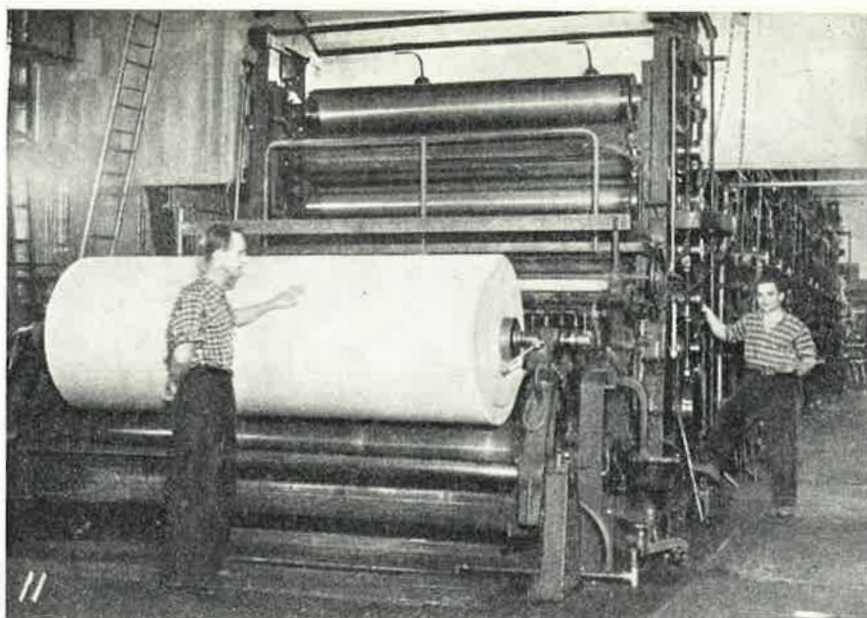
PK 5. Kalle Harju tunnustele paperiradan tasaisuutta Erkki Leipolan ollessa konekalanterin vieressä.
