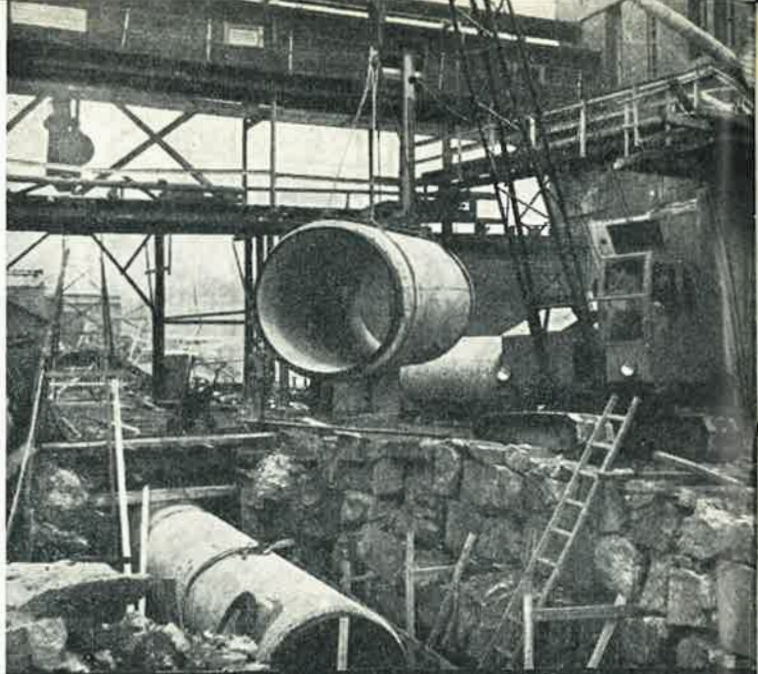
Lorain laskee Bonna-putken kaivantoon.
