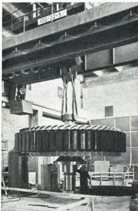
Siltanosturin koukussa riippuva juhllainen napapyörä on nostettu asennusaukon läpi konesaliin
