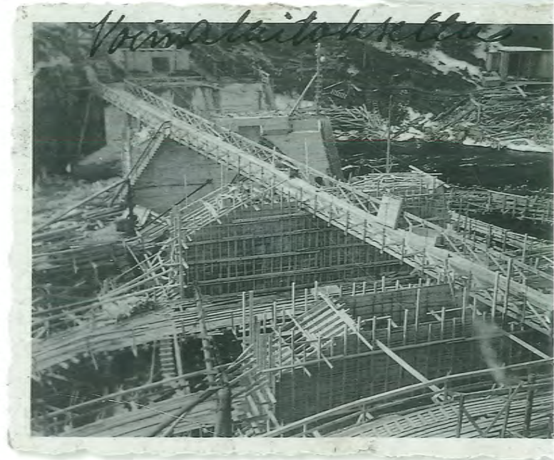
Keltin voimalaitoksen rakennuskuvia vuodelta 1939. Yläkuvassa Martti Mannisen työtovereita.
