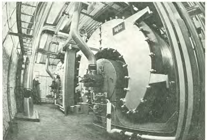
Heinolan tehdas on toimittanut Ruotsiin kaksi Högfors -42 kuumavesikattilaa, jotka tässä nähdään 'kalansilmäobjektiivin' läpi kuvattuna
