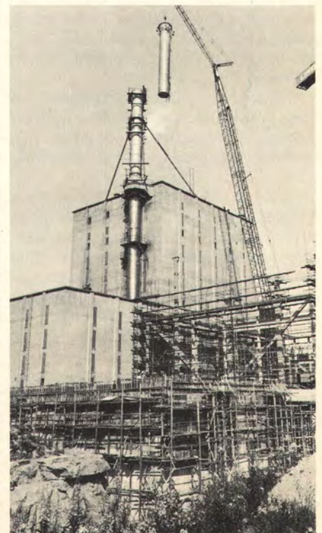
Kuusanniemen soodakattilavoimalaitoksen savupiippua pidennettiin Kuusanniemen rakennustöiden yhteydessä 17 metrillä. Vanha savupiippu katkaistiin juuresta, väliin asennettiin uusi osa ja vanha osa liitettiin piipun huipulle. Työn suoritti Götaverken.
