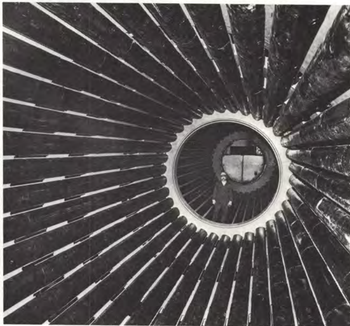
Heinolan tehtaalla Voikkaalle viime syksynä toimitettu kuorimarumpu ennen käynnistystä. Rummun halkaisija on 3,9 metriä ja pituus yhteensä 16 metriä.
