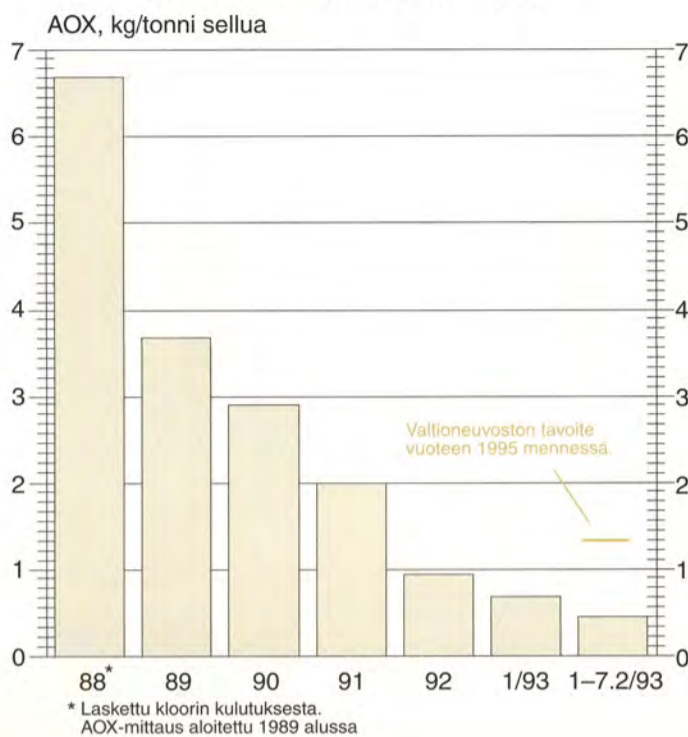
Kuusanniemen sellutehdas AOX-kuormitus 1988-1993
